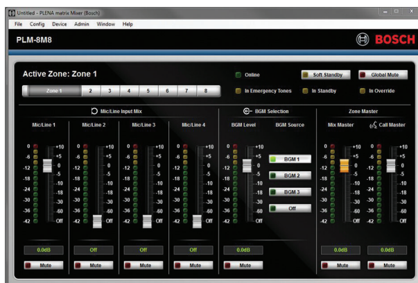
Рисунок 7.1: Главный экран графического интерфейса матричного микшера DSP
