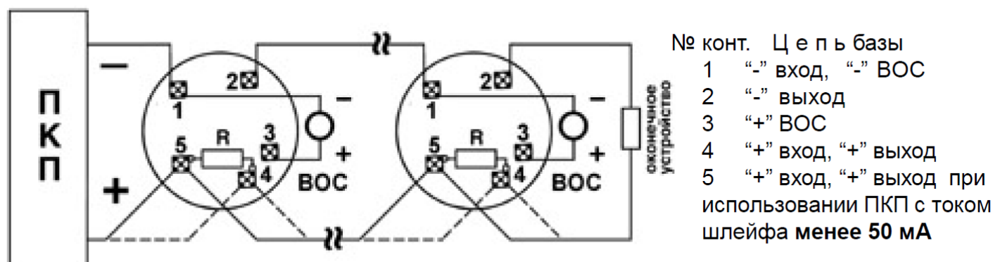
Рис.1. Схема подключения извещателей ИП212-58М с базами E1000R, E1000B к ПКП. Подключение с резистором показано пунктиром. В базе E1000B резистор и 4-й контакт не установлен.
