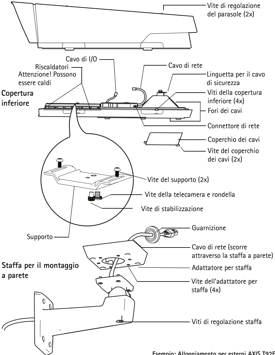
Esempio: Alloggiamento per esterni AXIS T92E20
