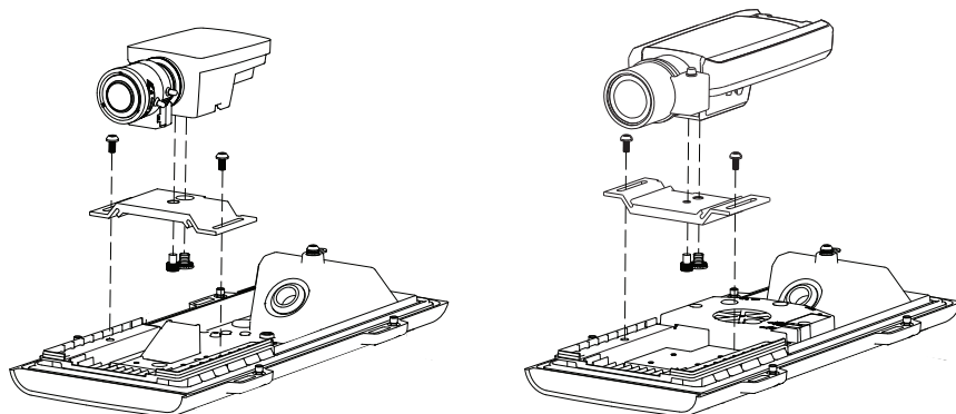
Exemples illustrés : Caméra réseau AXIS M1114 et caisson de protection AXIS T9E05 Caméra réseau AXIS P1343 et caisson d'extérieur AXIS T9E20
